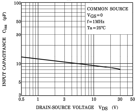
C_{iss} - V_{DS}
