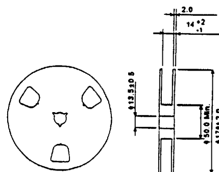
178 mm/7" Reel
